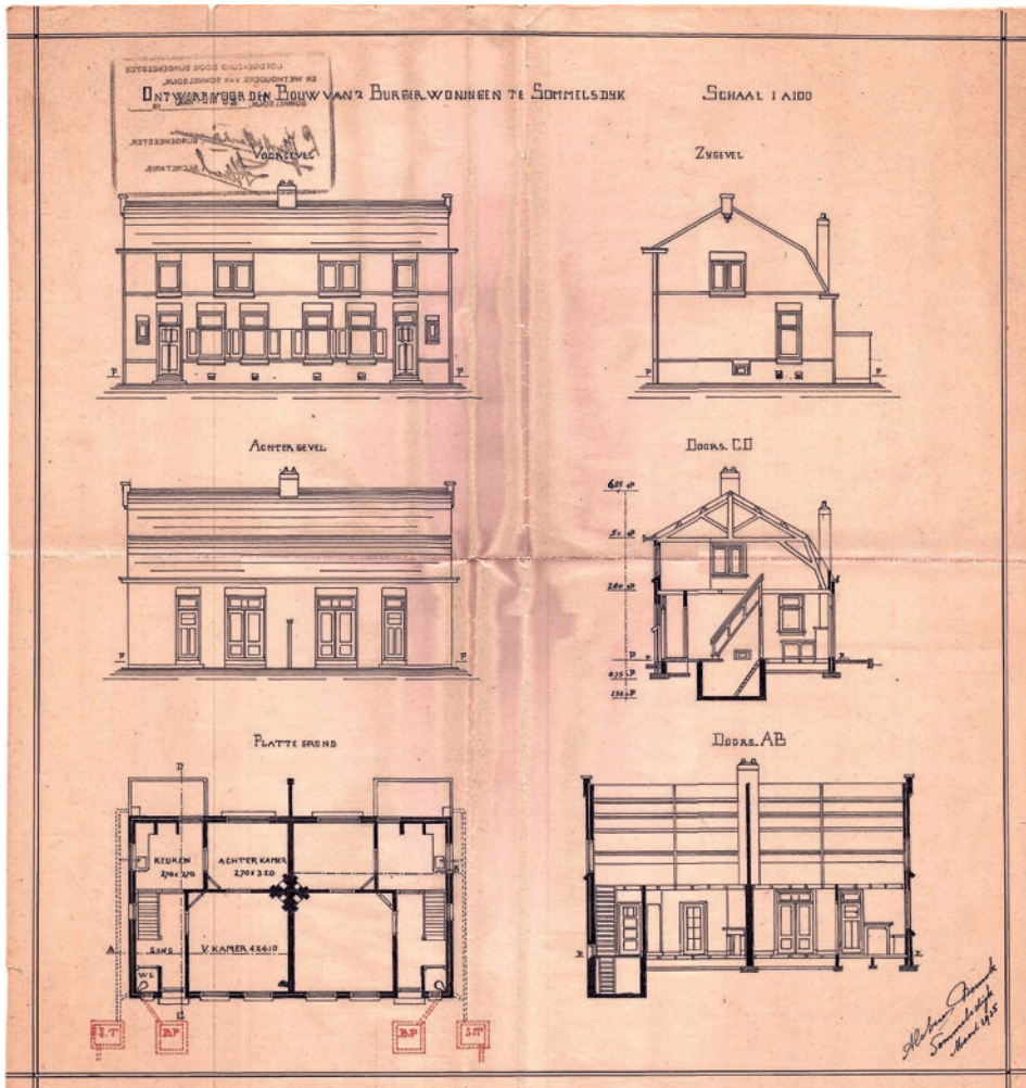
Bouwtekening voor de woningen van Mozes de Haas aan de Dorpsweg, 1936. 15
